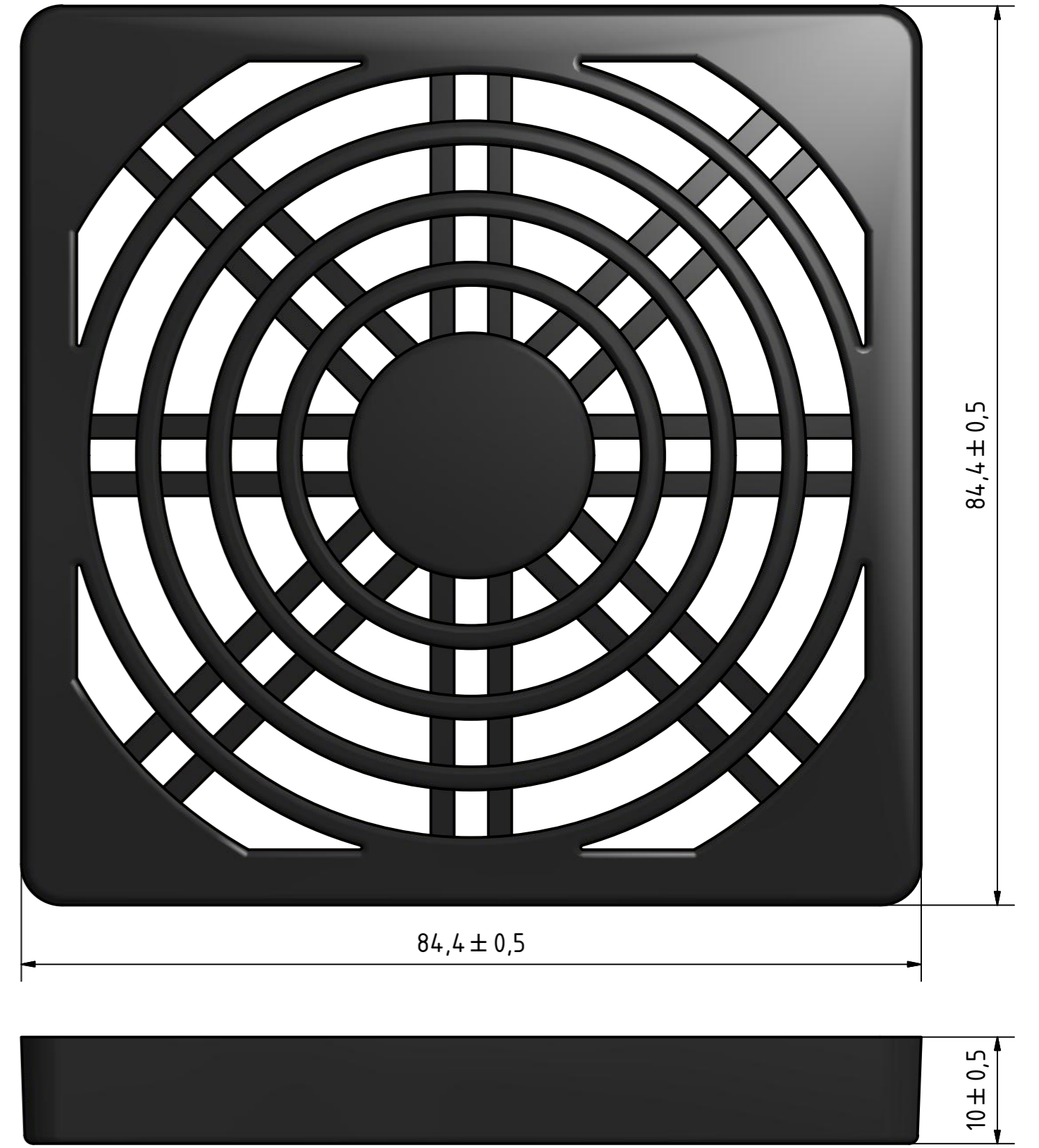
Außengitter
